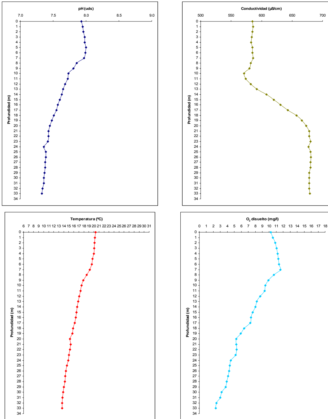
GRÁFICO 1 PERFILES FÍSICO-QUÍMICOS DEL EMBALSE DE CALANDA
